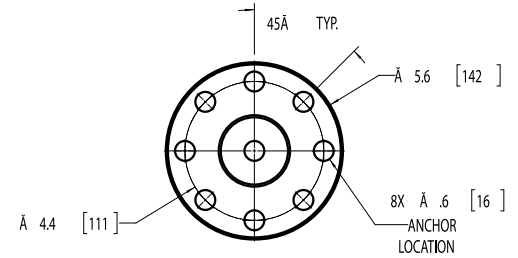
SECTION A-A SCALE 1:4
