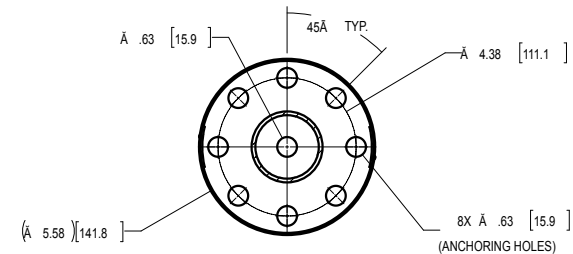
SECTION A-A SCALE 1 : 4
